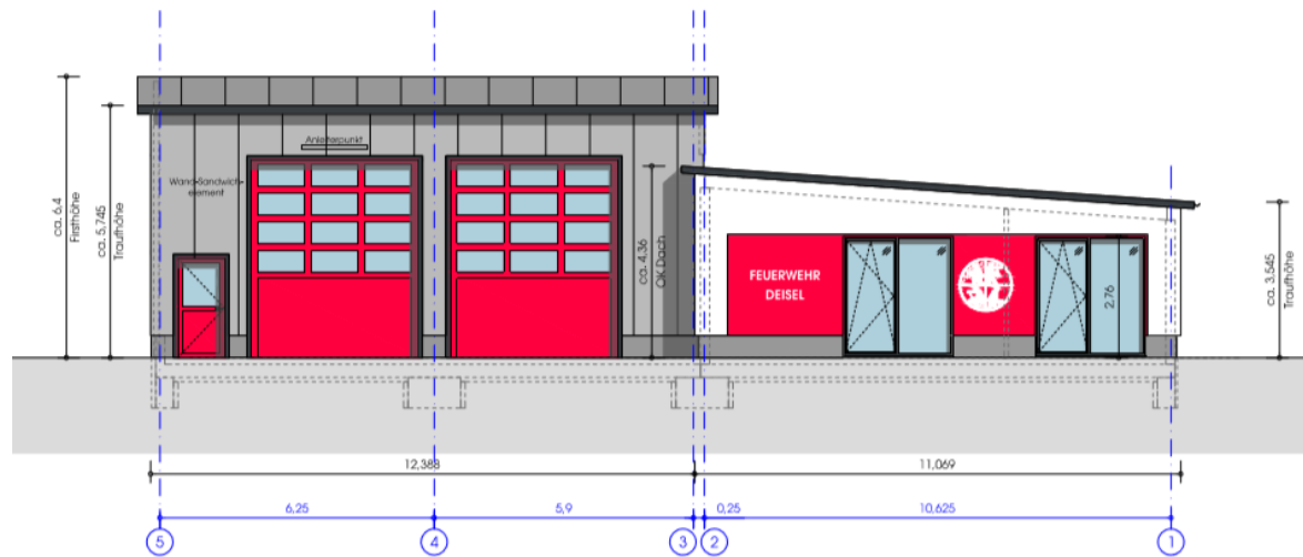
ht Nord-Ost | Fahrzeughalle + Sozialbereich | M 1:100
